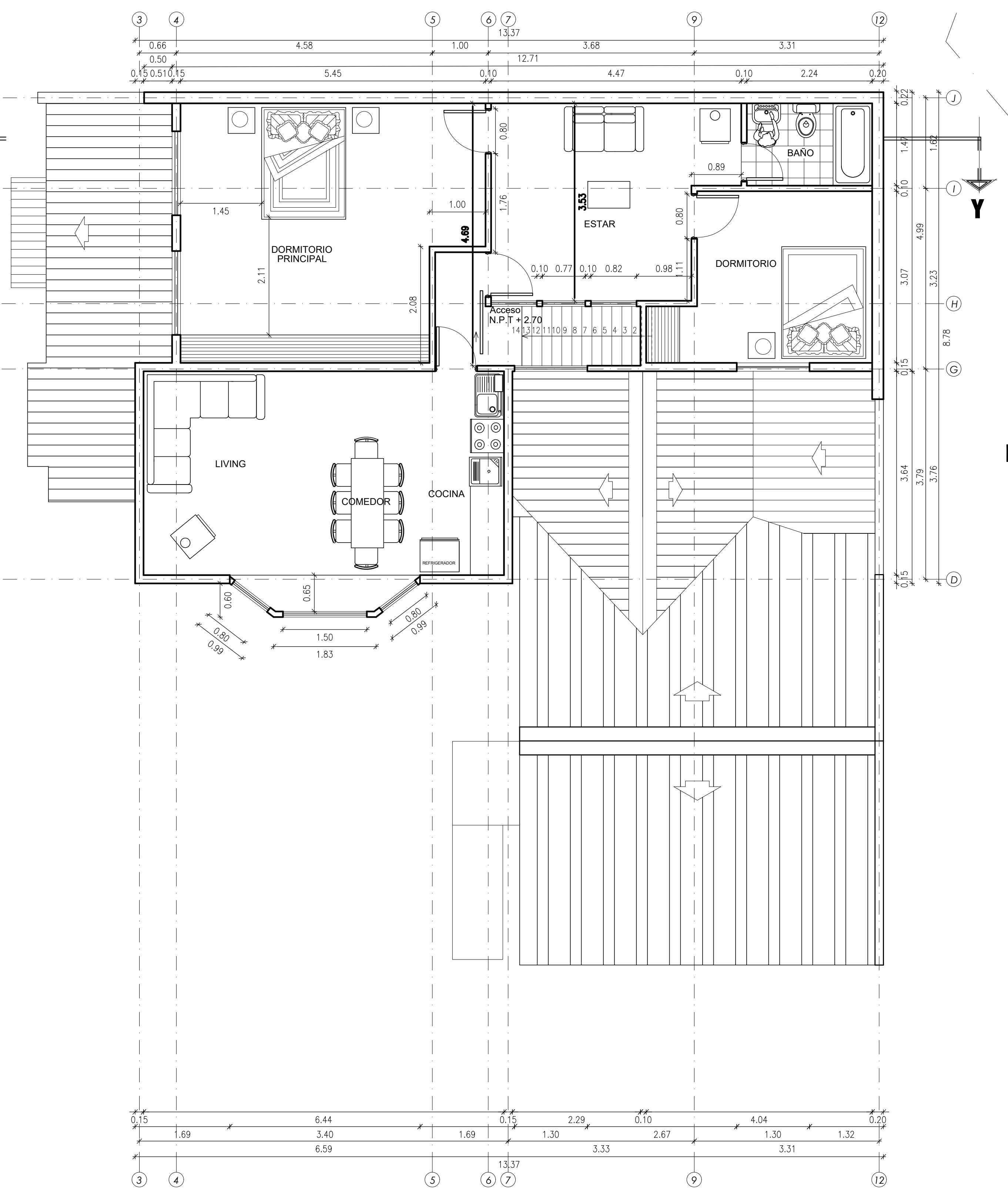
PLANTA ARQUITECTURA 2do NIVEL ESCALA 1/50
